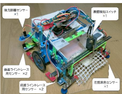
優勝したロボット「かっこす」
